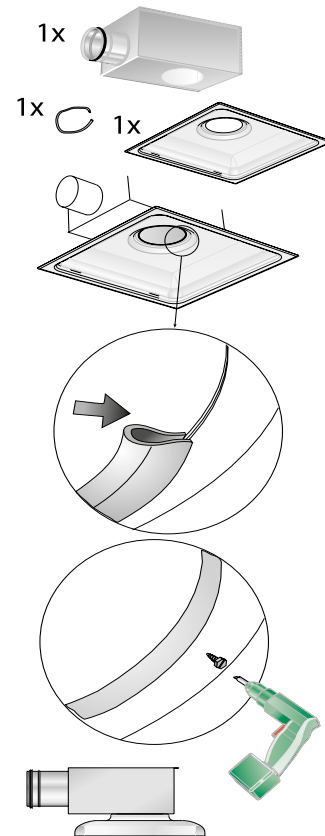
Abbildung 3. Montage von Luftauslass und Anschlusskasten bei geringer Bauhöhe.
