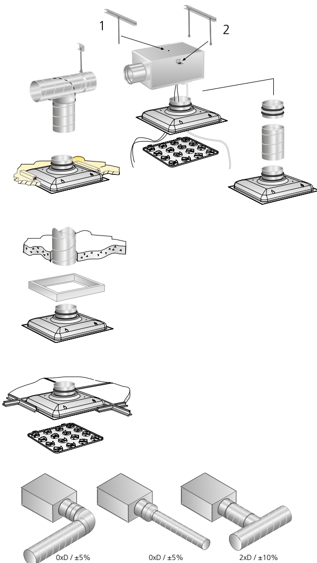
Abbildung 2. Montagealternativen.
