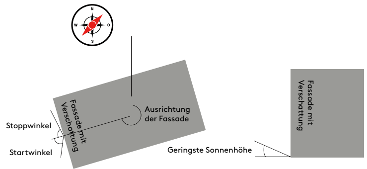
Einstellungen für die Fassade
