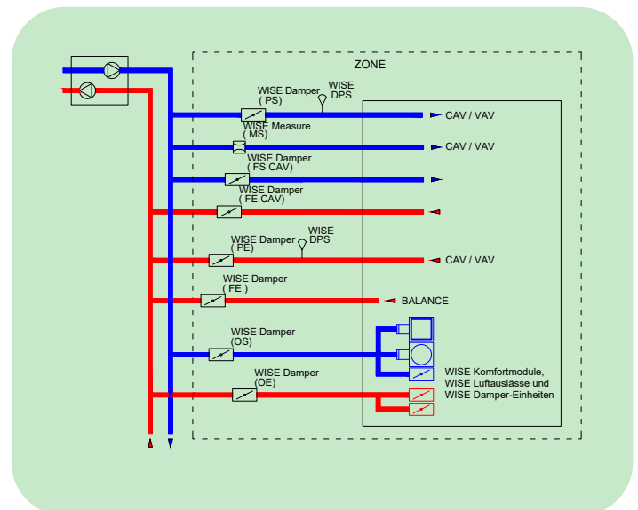
Prinzipische Schematische Darstellung, Volumenstromausgleich
