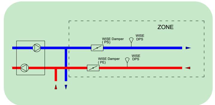
Prinzipische Skizze, Konstantdruckregelung
