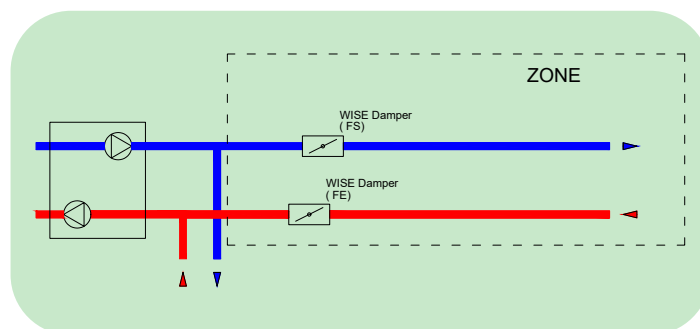
Prinzipiskizze, Konstantvolumenstromregelung
