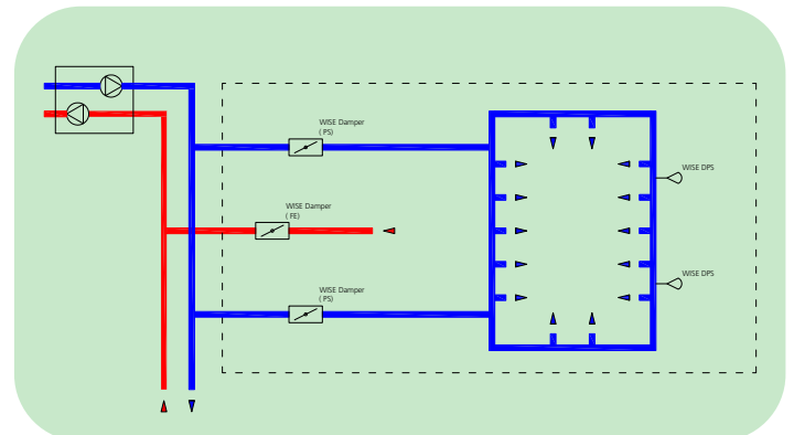
Prinzipialskizze, Gruppe für Konstantdruckregelung in ringgespeistem Kanalsystem
