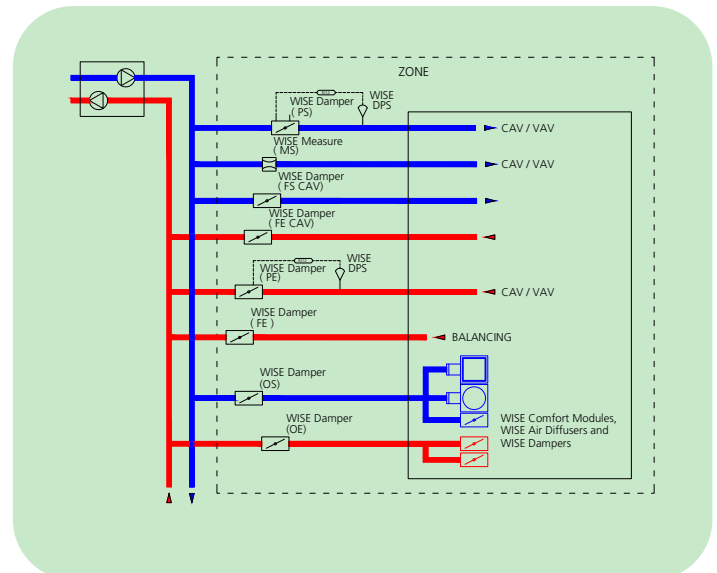
Schemat obwodu podstawowego, Równoważenie przepływu
