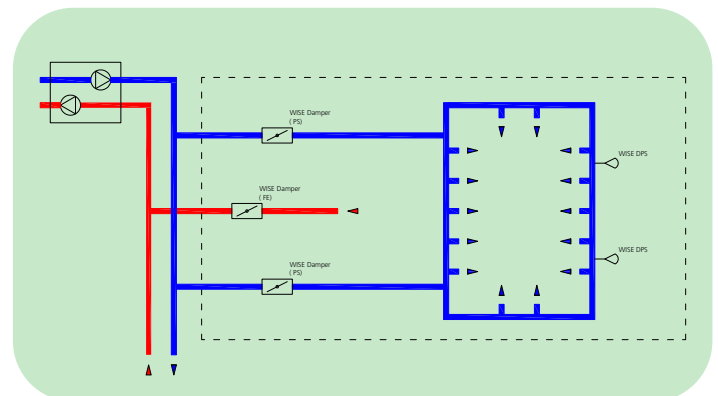
Schemat obwodu podstawowego: grupa stałej regulacji ciśnienia w „pierścieniowych” układach kanałowych
