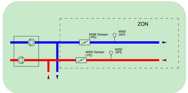
Schemat obwodu podstawowego, Regulacja ciśnienia stałego
