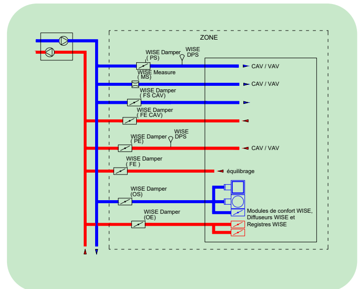
Schéma du circuit de base, équilibrage de débit
