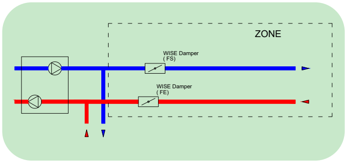
Schéma du circuit de base, régulation de pression constante
