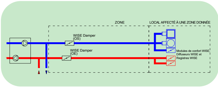
Schéma du circuit de base, optimisation de position
