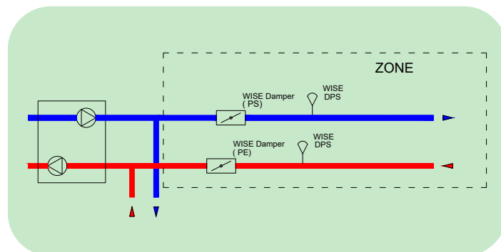
Schéma du circuit de base, régulation de pression constante
