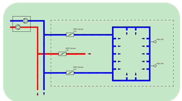
Schéma du circuit de base, groupe pour régulation de pression constante dans des systèmes de gaines alimentées en boucle
