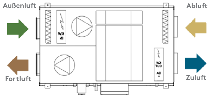
GLOBAL PX LP 02-04-06-08-10-14-18 (Ansicht von oben)
