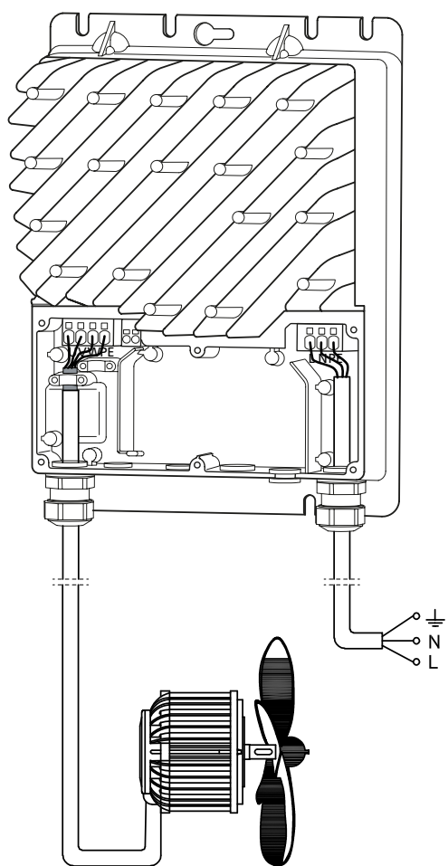
Abb. 7. Stromanschluss der Motorsteuerung, 0,8–1,5 kW.
