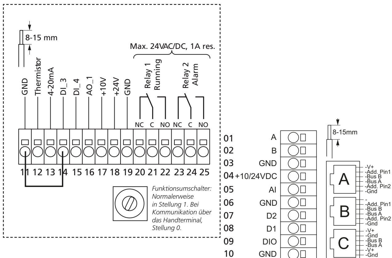
Abb. 1. Klemmen in der Motorsteuerung
