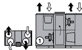
Zuluft unten (Links-Inspektion). Nicht RX Größe 004-008 in gemeinsamem Gehäuse.
