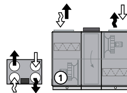
Zuluft unten (Links- Inspektion)
