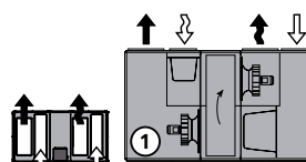
Zuluft unten (Links-Inspektion)
