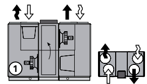
Abluft unten (Rechts-Inspek- tion). Nicht RX Größe 004-008 in gemeinsamem Gehäuse.
