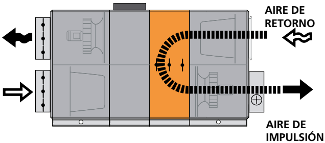
Calefacción nocturna intermitente con sección de recirculación:
