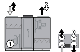
Aire de retorno hacia abajo (inspección hacia derechas)
