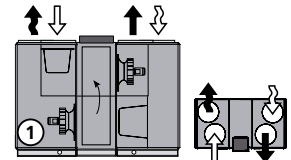
Aire de retorno hacia abajo (inspección hacia derechas). No hay RX tamaños 004-008 en caja común.
