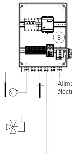
Compartiment Équipement 809535, unité de raccordement de tuyaux (accessoire, voir les instructions d'installation correspondantes)
