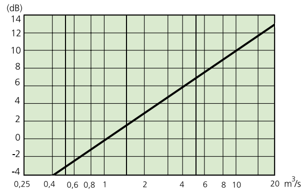
Diagramm 2. Korrektur für andere Luftvolumenströme als 1 \text{ m}^3/\text{s}
