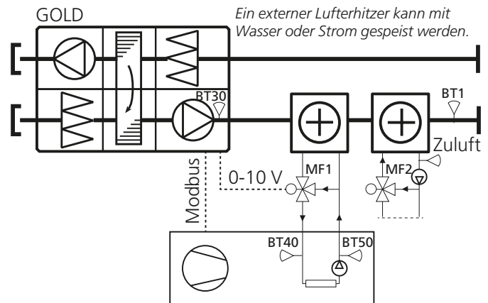
Swegon-Wärmepumpe Pumpe und Speichertank können hinzukommen und je nach Größe in oder neben der Wärmepumpe positioniert werden.
