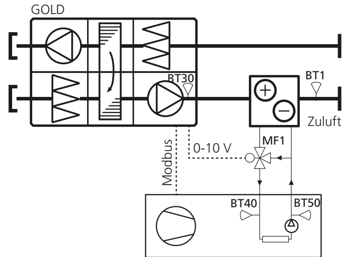
Swegon-Kältemaschine/ Wärmepumpe
