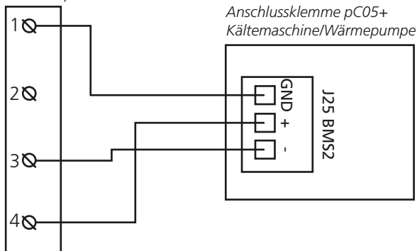
Anschlussklemme Kabeladapter TBLZ-64
