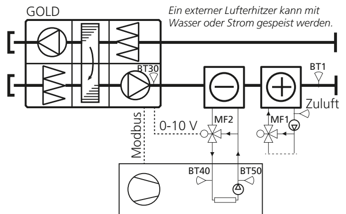
Swegon-Kältemaschine Pumpe und Speichertank können hinzukommen und je nach Größe in oder neben der Kältemaschine positioniert werden.
