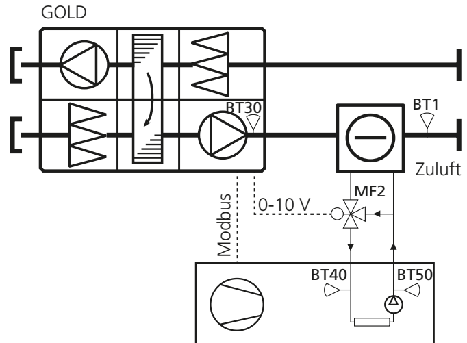
Swegon-Kältemaschine Pumpe und Speichertank können hinzukommen und je nach Größe in oder neben der Kältemaschine positioniert werden.
