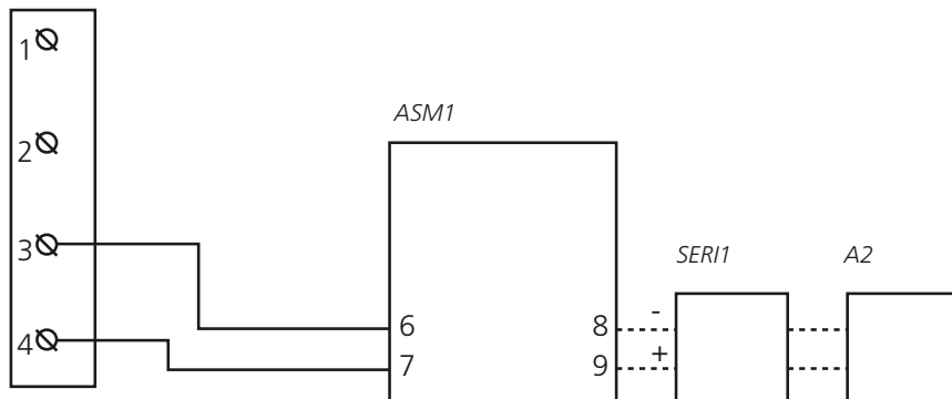
Anschlussklemme Kabeladapter
