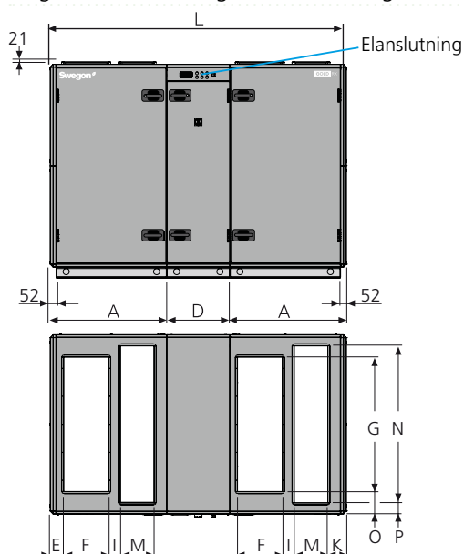
Vy ovanifrån. Visar aggregatets kanalslutningar för tilluftsfläkt höger uppe och vänster nere
