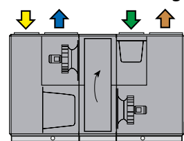
Tilluftsfläkt, vänster, uppe
