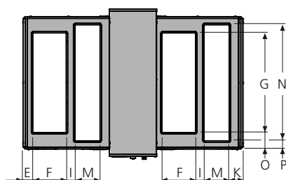
Vy ovanifrån. Visar aggregatets kanalslutningar för tilluftsfläkt höger uppe och vänster nere
