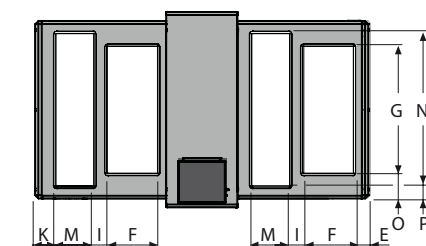
Vy ovanifrån. Visar aggregatets kanalslutningar för tilluftsfläkt höger nere och vänster uppe
