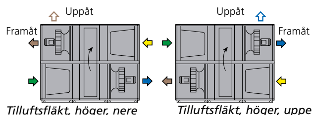
Högerutförande
