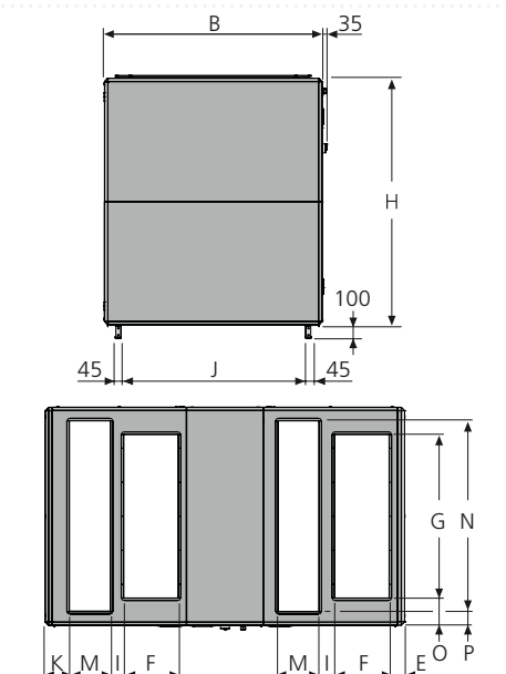
Vy ovanifrån. Visar aggregatets kanalslutningar för tilluftsfläkt höger nere och vänster uppe
