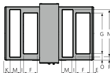
Vy ovanifrån. Visar aggregatets kanalslutningar för tilluftsfläkt höger nere och vänster uppe
