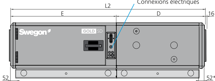
Ventilateur + batterie de récupération à eau glycolée
