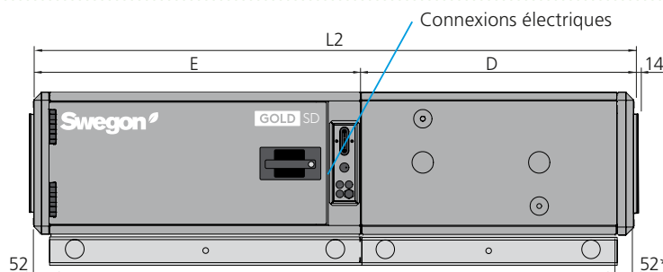
Ventilateur + batterie de récupération à eau glycolée
