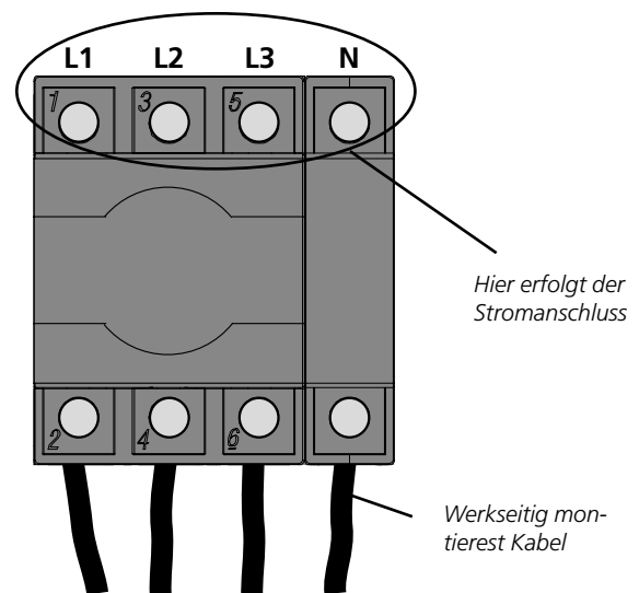
Block des Sicherheitsschalters.
