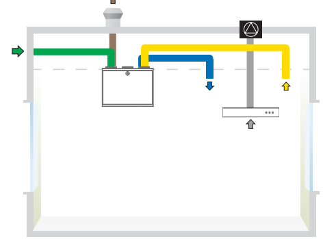
CASA W3 xs L Liesikupu liitettynä ulkoiseen huippumuriin.
