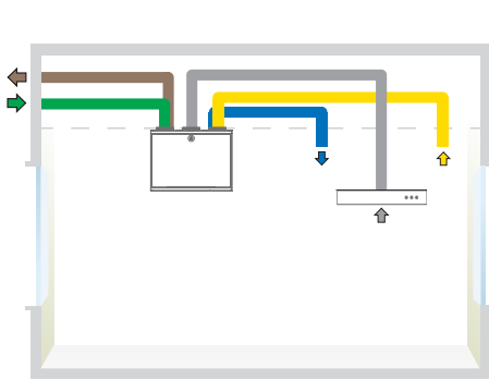
CASA W3 xs L Liesikupu liitettynä ilmanvaihdon keittiökanavayhteeseen.
