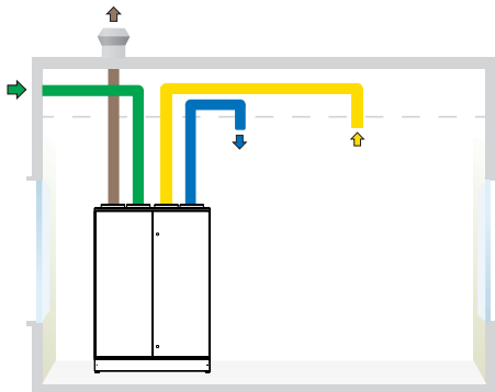
CASA W9 L Kanavaliitännät
