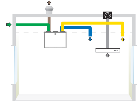
CASA W4 xs L Liesikupu liitettynä ulkoiseen huippumuriin.
