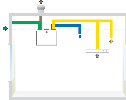
CASA W3 xs L Liesikupu liitettynä poistoilmakanavaan.
