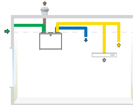
CASA W4 xs L Liesikupu liitettynä poistoilmakanavaan.
